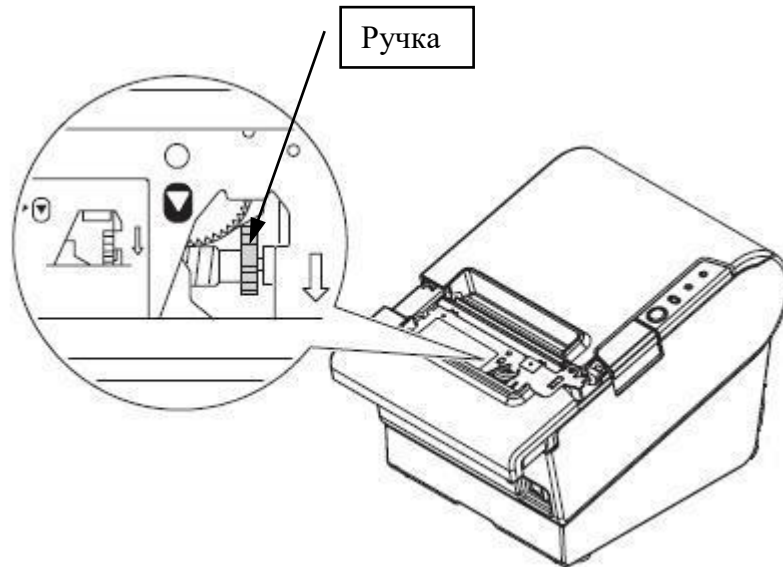
Рисунок 14 – Налаштування нормального положення леза обрізувача.
