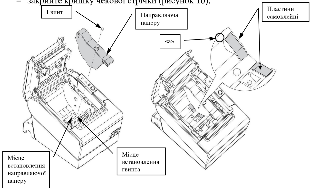
Рисунок 12 – Зміна ширини паперу
