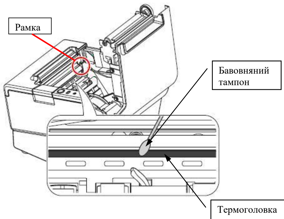
Рисунок 15 – Очистка термоголовок реєстратора.
