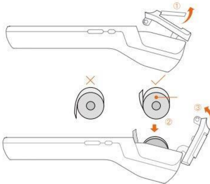
Рисунок 3.1 – Встановлення паперової стрічки
